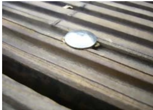
Einfache Lösung: Schlossschraube versenkt sich ohne Gummi von selbst
